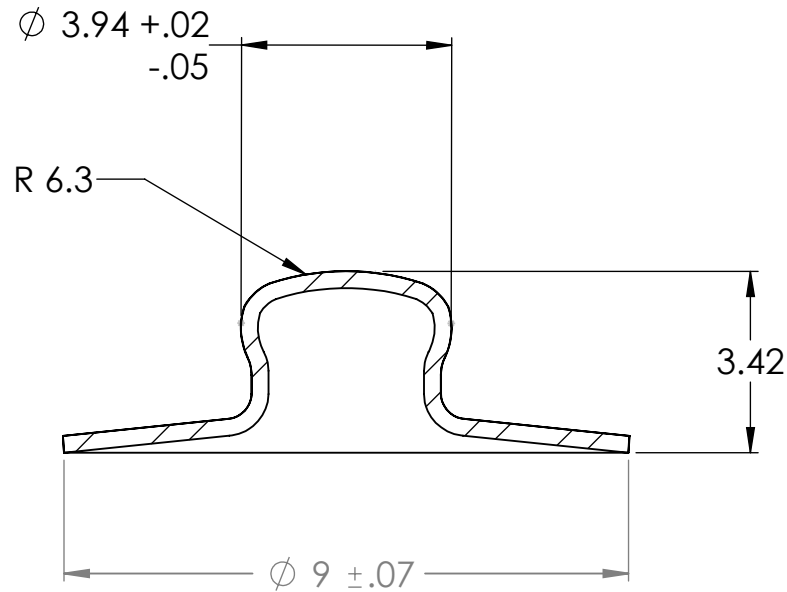
SECTION A-A SCALE 7 : 1
