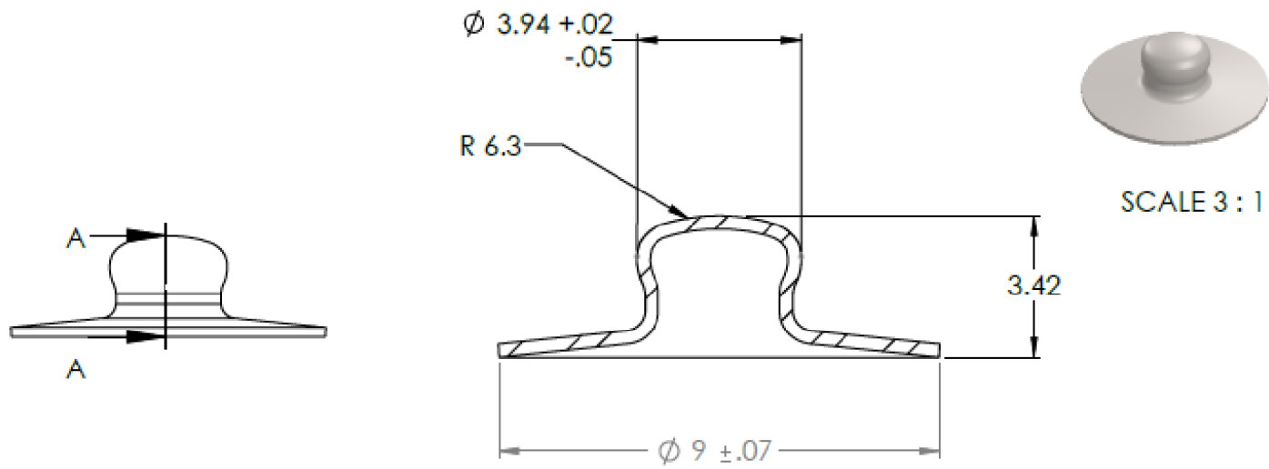
SECTION A-A SCALE 7 : 1
